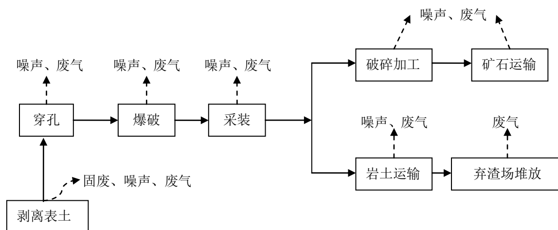
图 5-2 生产工艺流程图
